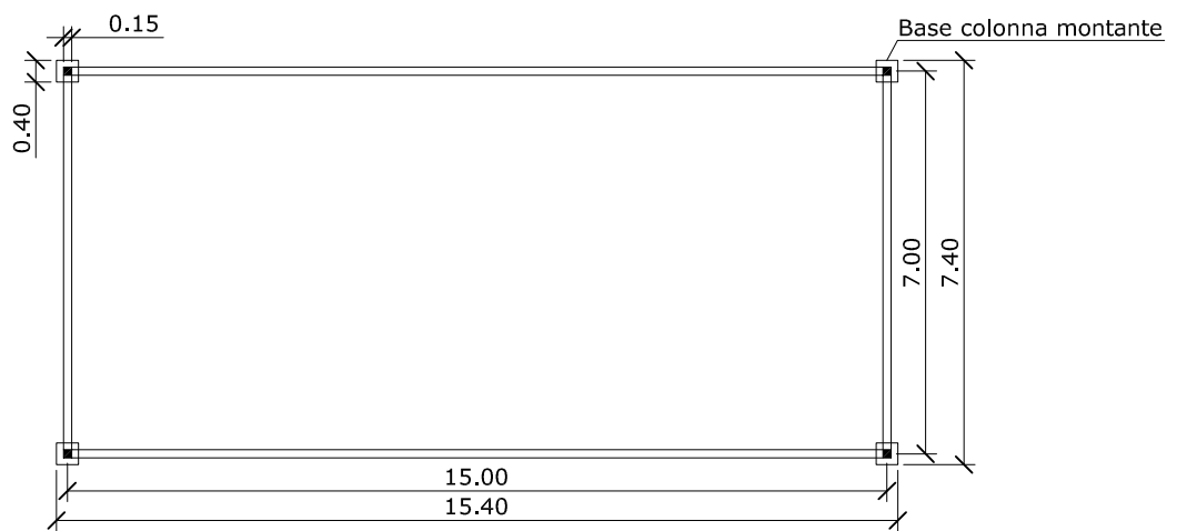
- PIANTA
