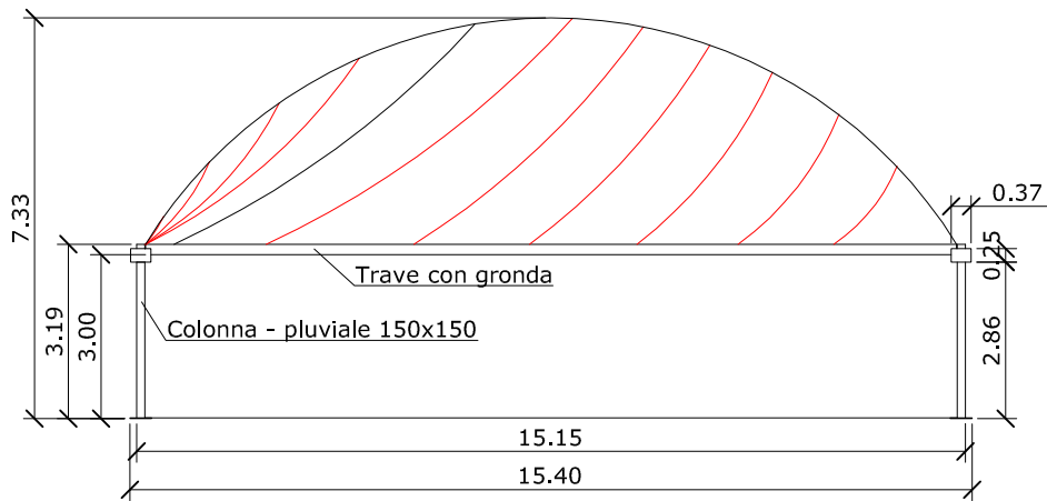
- PROSPETTO
